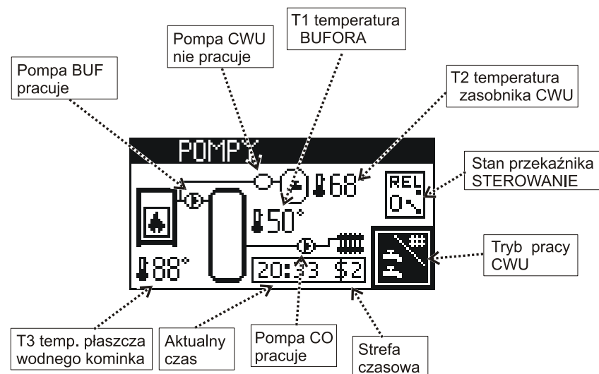
Ekran pracy pomp dla alternatywnego układu pracy (CWU przed BUF)
