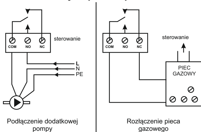
Rys.4 Schemat wykorzystania styku STEROWANIE
