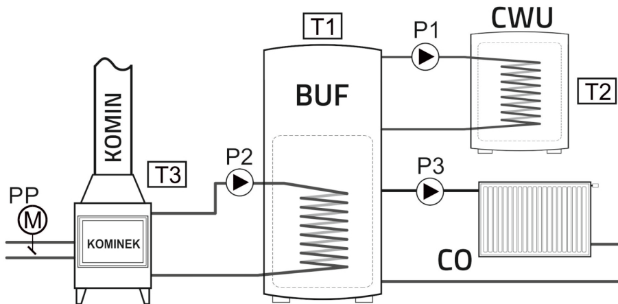
Rys.1a Podstawowy układ pracy regulatora (CWU za BUF). Parametr „<93> CWU przed BUF”=WYŁ.
