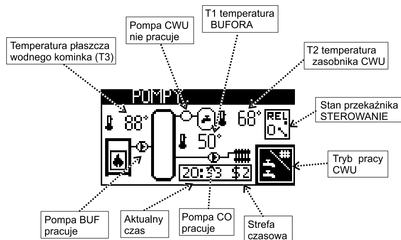
Ekran pracy pomp dla podstawowego układu pracy (CWU za BUF).
