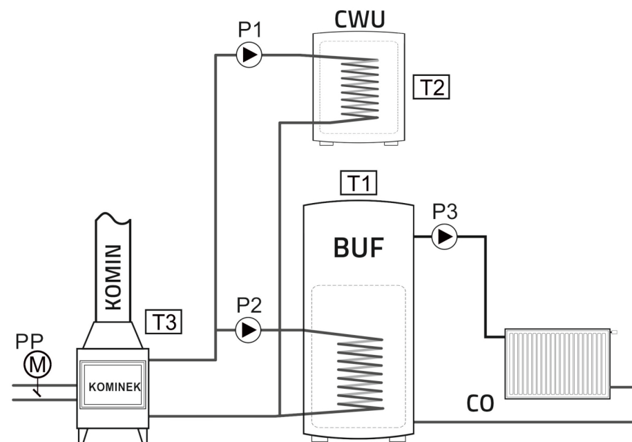
Rys.1b Alternatywny układ pracy – (CWU przed BUF). Parametr „<93> CWU przed BUF”=ZAŁ.
