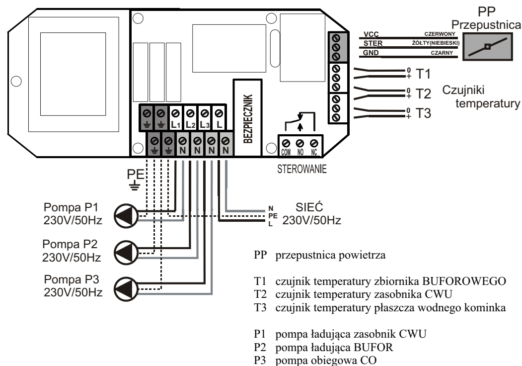
Rys.3 Schemat instalacji elektrycznej
