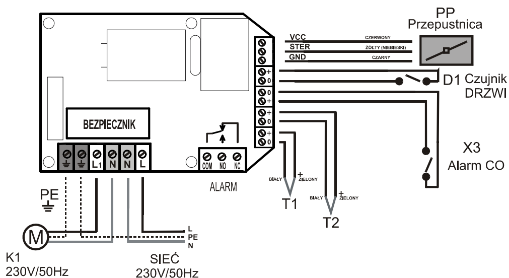
Rys.3 Schemat instalacji elektrycznej
